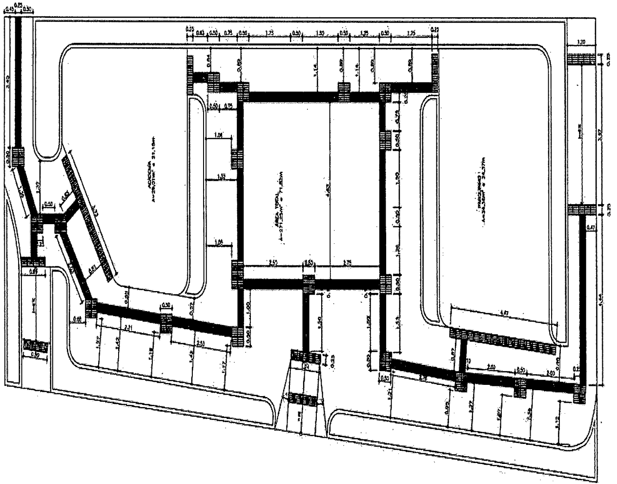
PISO TÁTIL - SERRA Esc. 1/50
